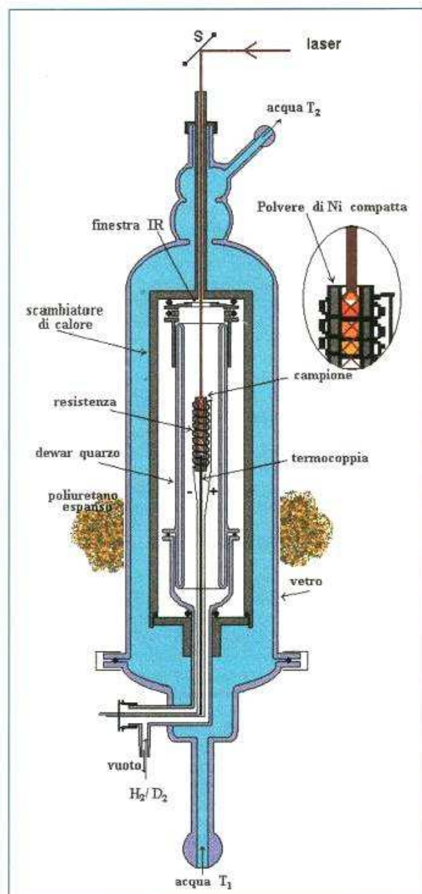
Cella calorimetrica a flusso d'acqua
